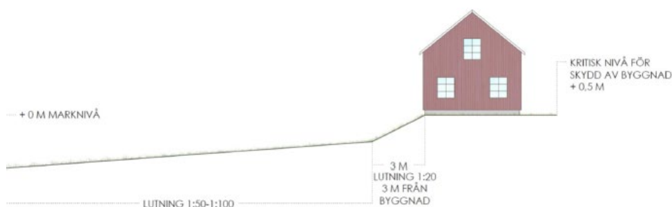
Principskiss för höjdsättning (Norconsult Sverige AB)
